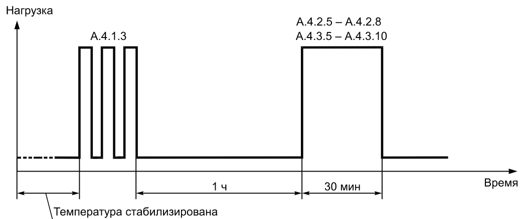
Рисунок А.2 — Рекомендованная последовательность испытаний для каждой температуры при определении невозврата выходного сигнала при возврате к минимальной нагрузке DR и испытаниях на ползучесть при выполнении испытаний в устройстве, отличающемся от того, в котором проводились испытания под нагрузкой
